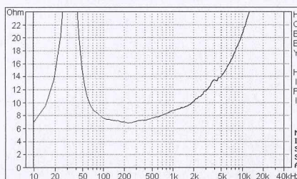
Relativ niedrige Schwingungspuleninduktivität, Resonanzzeichen bei 4 kHz.
